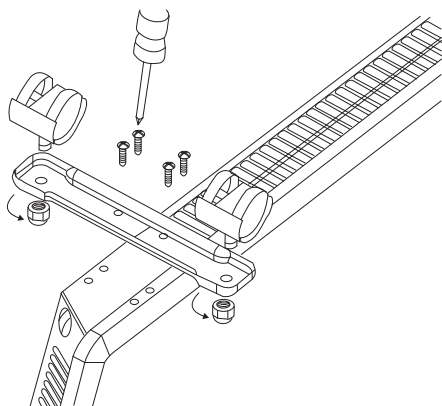
Рис. 6. Ножка
